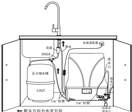
安装于橱柜下 根据您家庭厨房具体的布置情况安装在橱柜下。 注：请专业技术人员安装。
